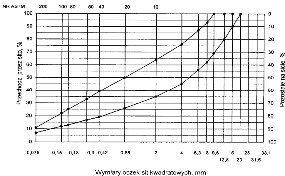
Wymiary oczek sit kwadratowych, mm Rys. 1. Krzywe graniczne uziarnienia mieszanki mineralnej BA od 0 do 20 mm do warstwy ścieralnej nawierzchni drogi o obciążeniu ruchem dla KR1 lub KR2
