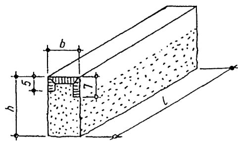
Krawężnik uliczny rodzaju B
