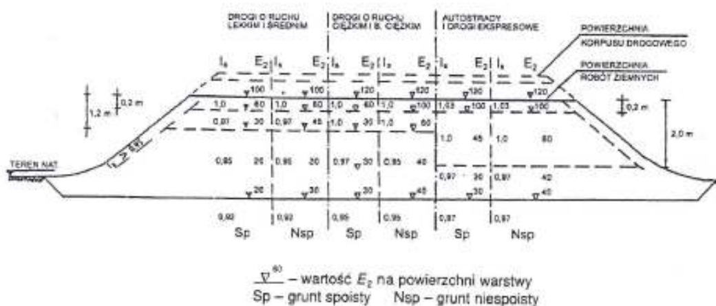
Rysunek 3 – Wartości wymagane w nasypach: Wskaźnika zagęszczenia I_k i wtórnego modułu odkształcenia E_2 , megapaskali
