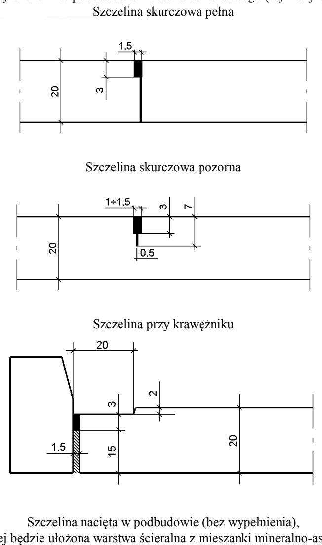
Rys. 1.1. Przykłady konstrukcji szczelin w podbudowie z betonu cementowego (wymiary w cm)
