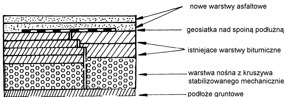
Rys. 5. Wzmocnienie nawierzchni asfaltowej w strefie poszerzenia nawierzchni a) wariant 1
